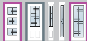
090 (3x) 23" x 18" 104 23" x 49" 105 9" x 49" 107 8" x 65" 108 23" x 65"
